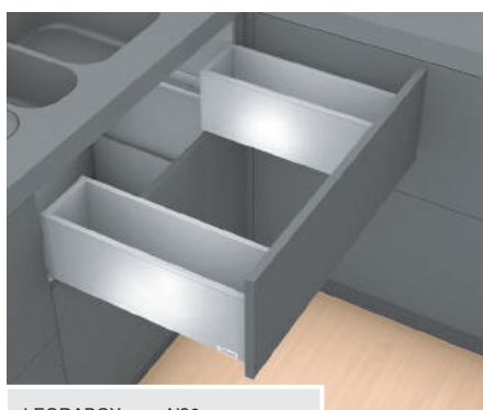
LEGRABOX pure №9
